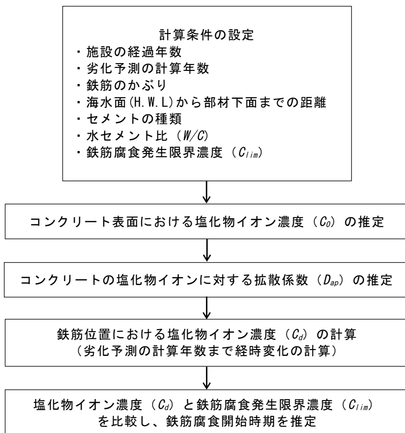
図 3-3.6 塩化物イオンの浸透による鉄筋腐食の開始時期の予測の基本的な手順
