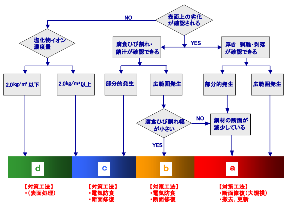
図 3-3.11 劣化度を目安とした対策工法の選定フロー (手引き)
