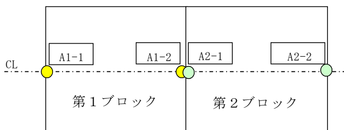
図 3-4.4 位置座標の測点例（ケーソン式防波堤）
