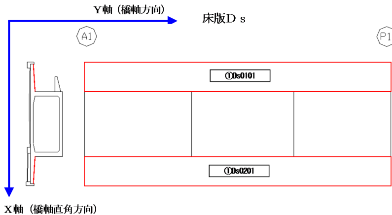
図 3-4. 14 床版に対する座標系
