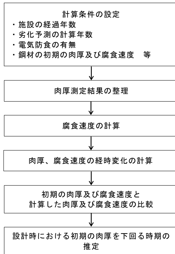
図 3-3.7 鋼材の肉厚及び腐食速度の予測の基本的な手順
