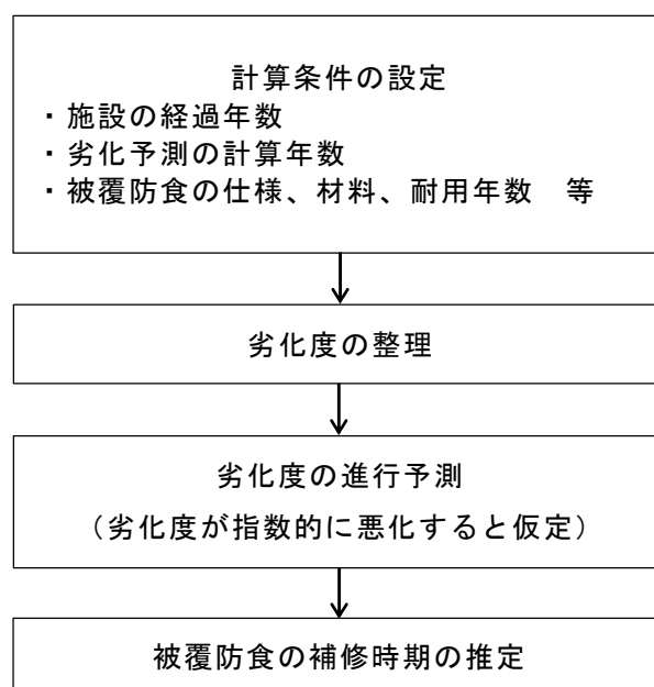
図 3-3.9 耐用年数に基づく被覆防食工の劣化予測の基本的な手順
