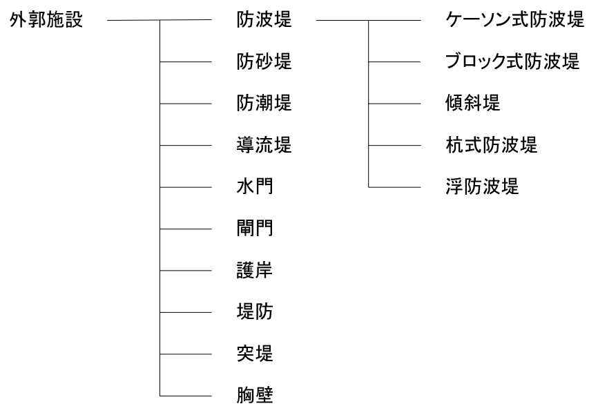
図 3-4.2 外郭施設の種類及び代表的な構造形式
