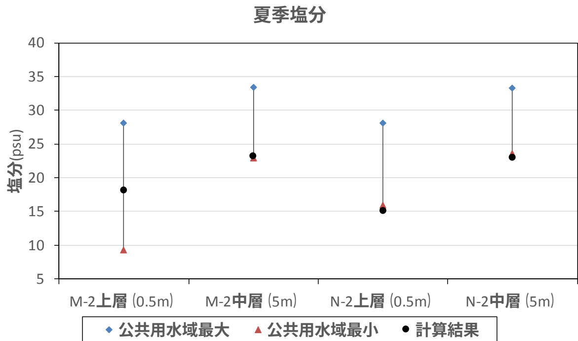
図 7-4-11 愛知県公共用水域水質調査地点における水温・塩分の比較（夏季）
