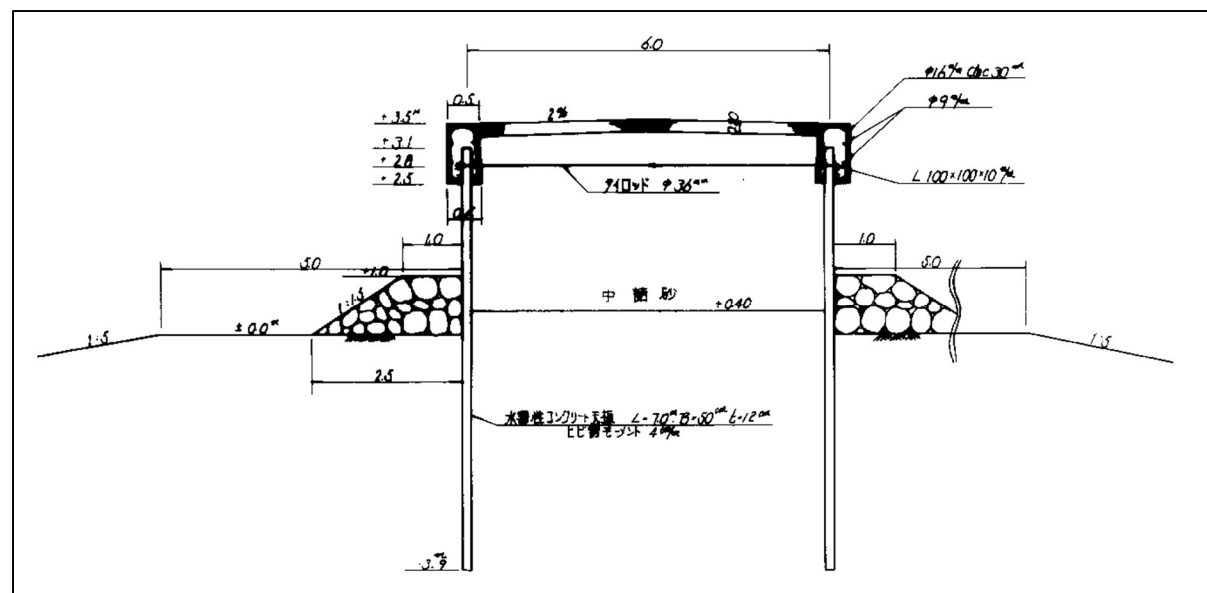
地骨標準断面図（上部アスファルト部分は撤去済）
